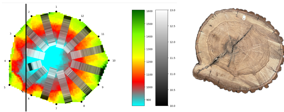
Figura 3: A la izquierda, la combinación de datos del resistógrafo y el tomógrafo en una herramienta que permite desplazar la superposición de imágenes para facilitar su interpretación. A la derecha, el estado real de la sección transversal del tronco obtenida tras la tala. La foto demuestra que no había cavidad en el árbol, sino una grieta en los puntos donde la perforación entre los sensores 4 y 5 la reveló. Observe la caída en la curva y el punto negro en la columna correspondiente con niveles de gris. (Foto V. Semík)
