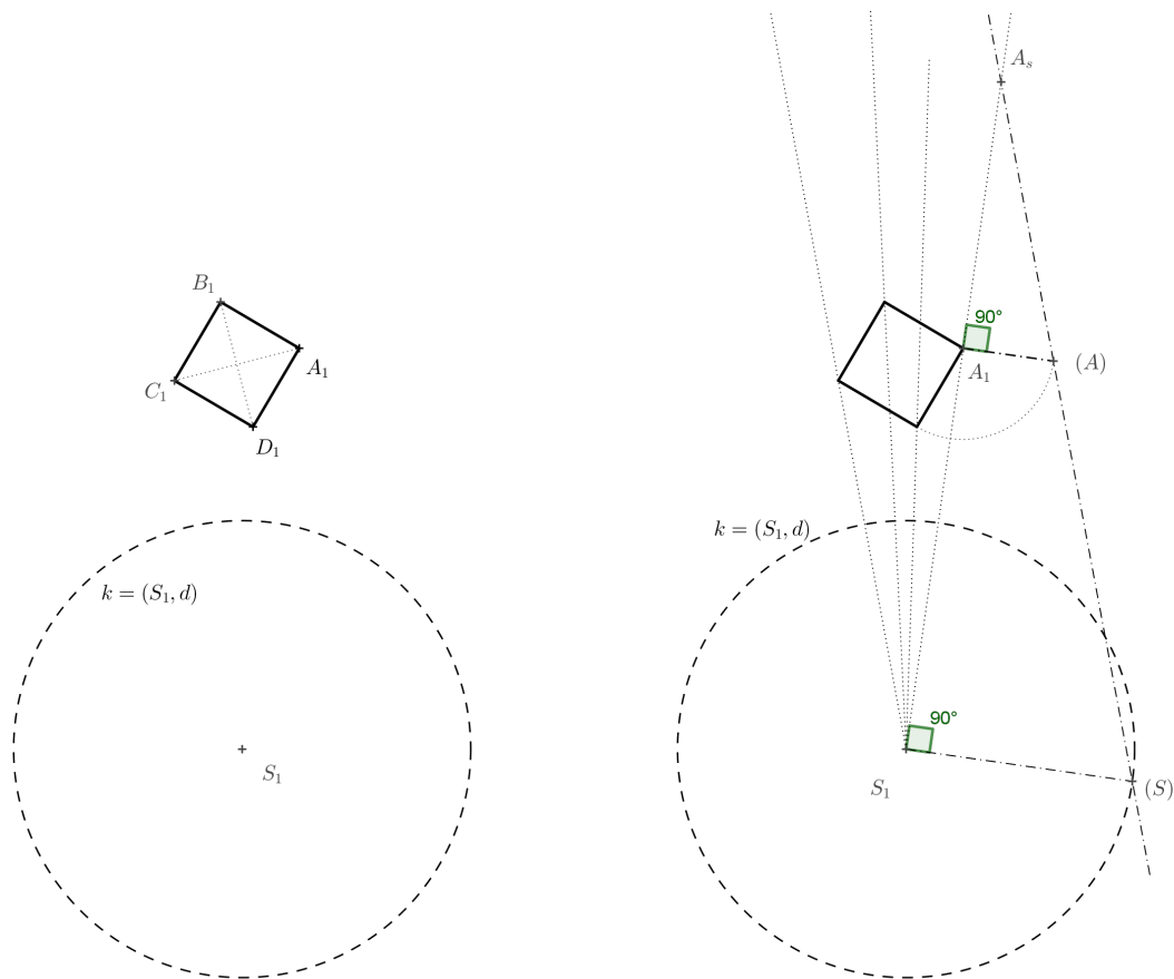
Obrázek 9: Zobrazení čtverce dolní podstavy a určení bodu A_s
