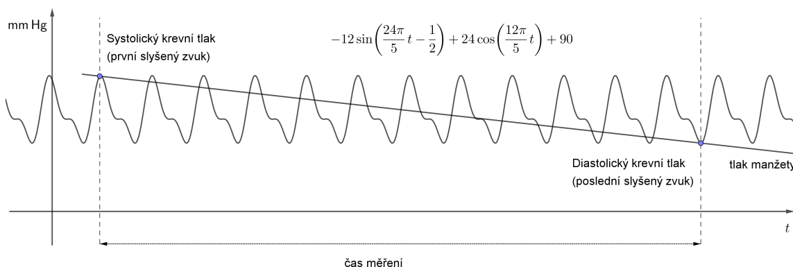
Obrázek 2: Příklad součtu sinu a kosinu s různými periodami
