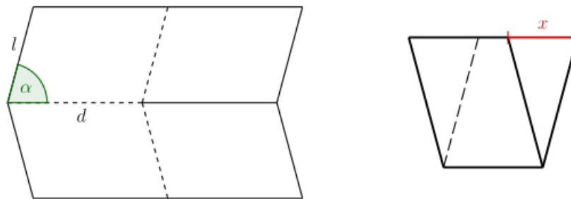
Obrázek 7: Základní část vzoru Miura Ori v rozloženém a složeném stavu
