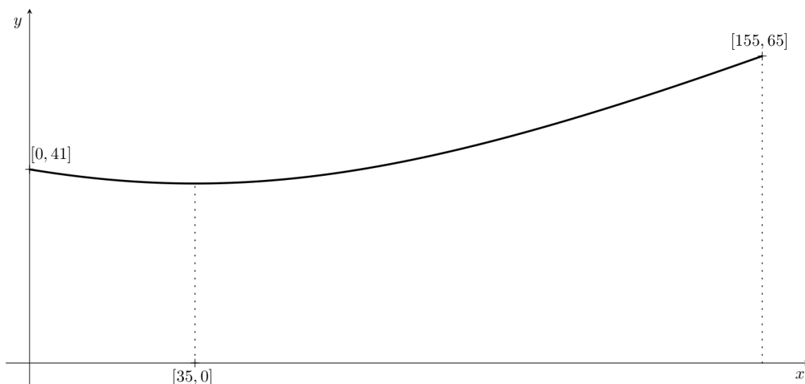
Rysunek 2: Przekrój poziomej wieży chłodniczej. Korona wieży znajduje się po lewej stronie, a podstawa po prawej.
