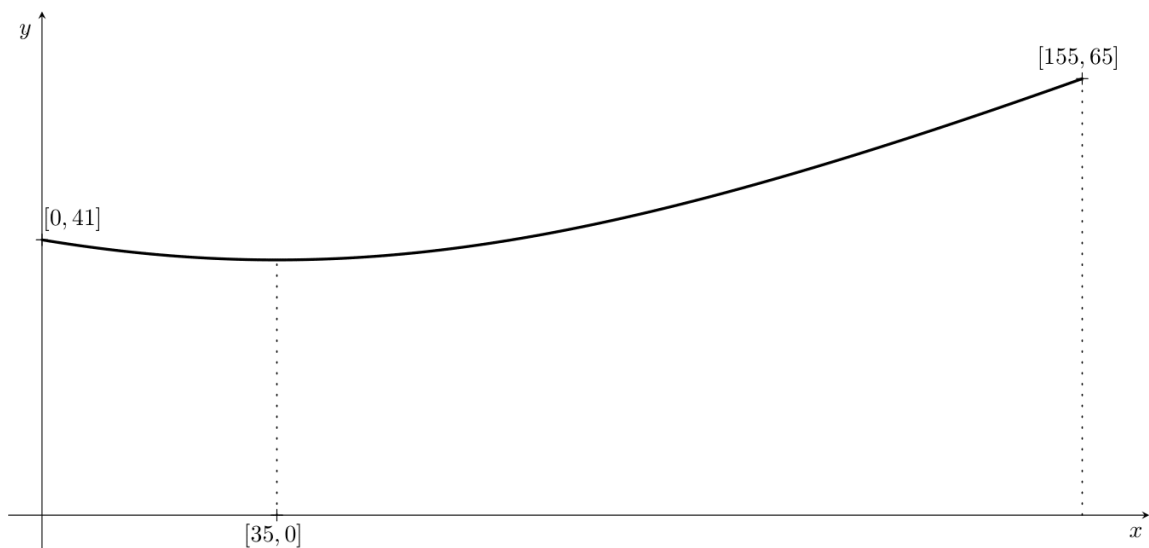
Obrázek 2: Řez ležící chladící věže. Koruna věže je umístěna vlevo, základna vpravo
