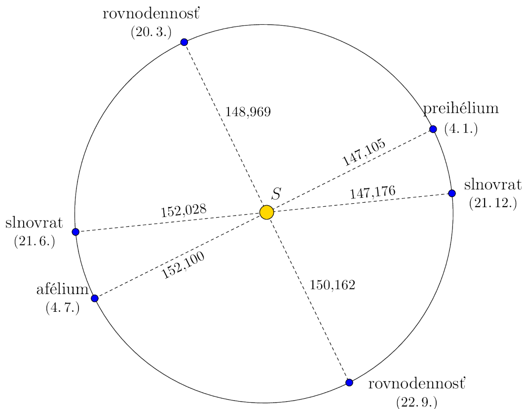
Obr. 3: Trajektoría Zeme okolo Slnka v mierke
