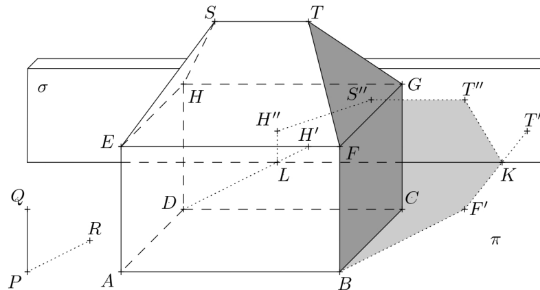
Rysunek 3: Odlew i cień własny całego domu ze ścianą
