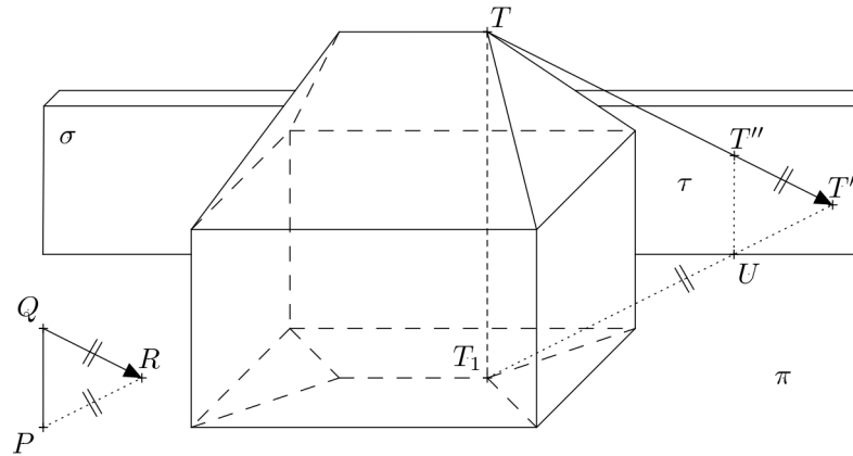
Rysunek 2: Konstruowanie rzucanego cienia punktu za pomocą ściany
