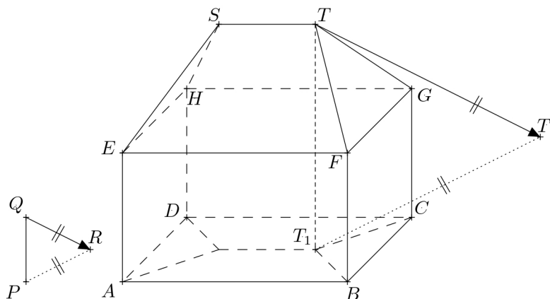
Rysunek 1: Konstruowanie rzucanego cienia punktu T
