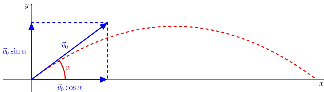
Obrázek 1: Šikmý vrh
